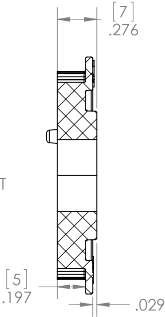
SECTION A-A
